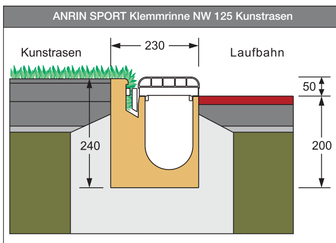
ANRIN SPORT Entwässerungssystem NW 125 Kunstrasen Klemmrinne NW 125 für Kunstrasenspielfelder in Kampfbahnen Typ A bis D. Spielfeldüberhöhung gegenüber Laufbahn ca. 5 cm
